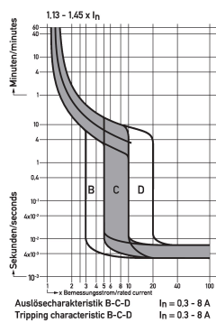
Diagramme Leitungsschutzschalter DLS 6i Co6-1
