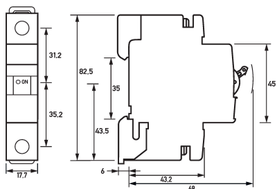
Maßzeichnung Leitungsschutzschalter DLS 6i Co6-1
