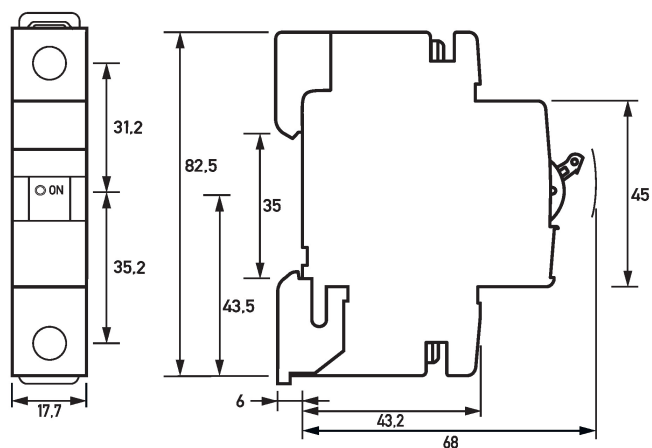
Maßzeichnung DLS 6i, C-Charakteristik, einpolig, 10kA (Gruppenansicht)
