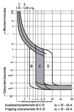
Diagramas Interruptores magnetotérmicos DLS 6i B40-3+N
