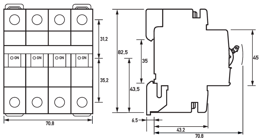
Maßzeichnung DLS 6i, B-Charakteristik, dreipolig+N, 10kA (Gruppenansicht)
