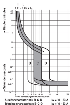
Diagrams miniature circuit-breakers DLS 6i B16-2
