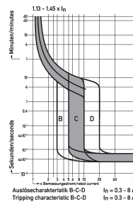
Curva característica Característica B, C, D
