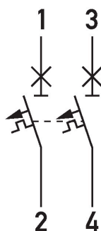
Anschlussschema DLS 6i, B-Charakteristik, zweipolig, 10kA
