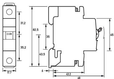
Maßzeichnung Leitungsschutzschalter DLS 6i B40-1
