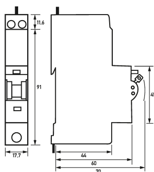
Dibujo acotado Combinaciones de interruptores diferenciales e interruptores magnetotérmicos RCBO 1 C25/0,03/1-AC
