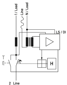
Ejemplo de cableado Combinaciones de interruptores diferenciales e interruptores magnetotérmicos RCBO 1 C25/0,03/1-AC
