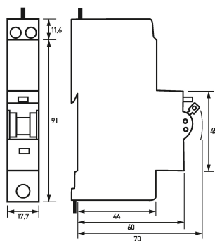
Dibujo acotado Combinaciones de interruptores diferenciales e interruptores magnetotérmicos RCBO 1, tipo AC, 1 polo
