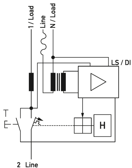
Anschlussschema RCBO 1, Typ AC, 1-polig
