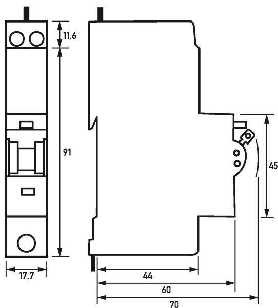
Maßzeichnung RCBO 1, Typ AC, 1-polig (Gruppenansicht)
