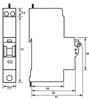
Dibujo acotado Combinaciones de interruptores diferenciales e interruptores magnetotérmicos RCBO 1 C13/0,03/1-A
