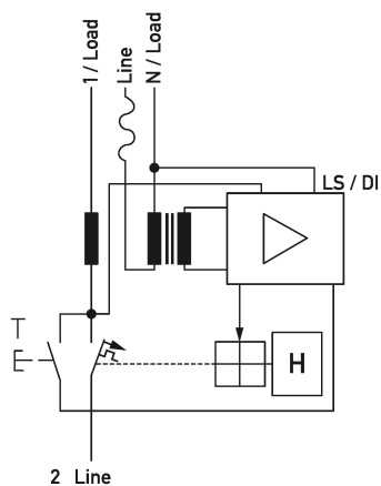
Esquema de conexiones RCBO 1, tipo A, 1 polos
