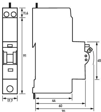
Dibujo acotado RCBO 1, tipo A, 1 polos (Vista de grupos)
