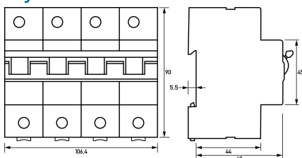
Maßzeichnung Gruppenansicht
