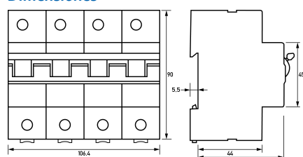
Dibujo acotado Vista de grupos
