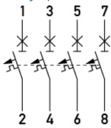
Anschlussschema
