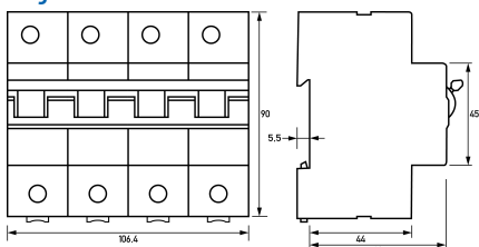
Maßzeichnung Gruppenansicht
