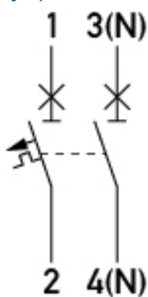
Esquema de conexiones
