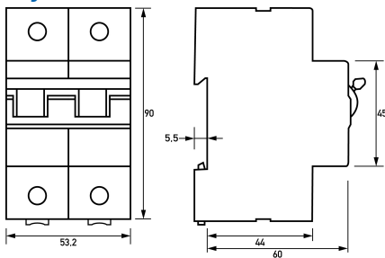
Maßzeichnung Gruppenansicht
