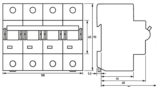
Dibujo acotado Interruptores magnetotérmicos DMCB 2 C125-3N
