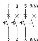
Ejemplo de cableado Interruptores magnetotérmicos DMCB 2 C125-3N
