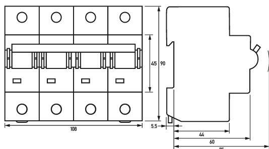
Dibujo acotado Interruptores magnetotérmicos DMCB 2 C100-4
