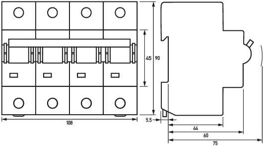
Dibujo acotado Interruptores magnetotérmicos DMCB 2 Co80-4
