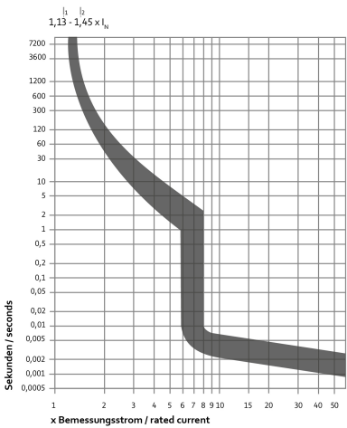
Diagramas Interruptores magnetotérmicos DMCB 2 Co80-4
