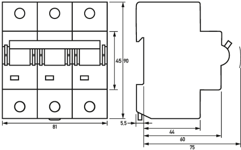
Dibujo acotado Interruptores magnetotérmicos DMCB 2 C100-3
