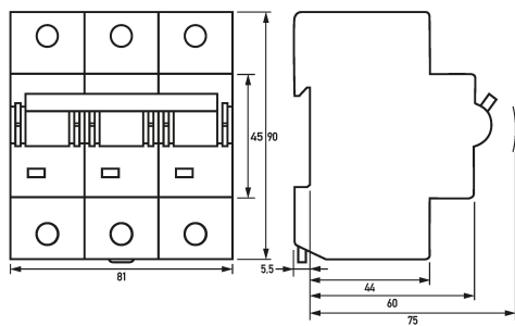
Dibujo acotado Interruptores magnetotérmicos DMCB 2 Co80-3
