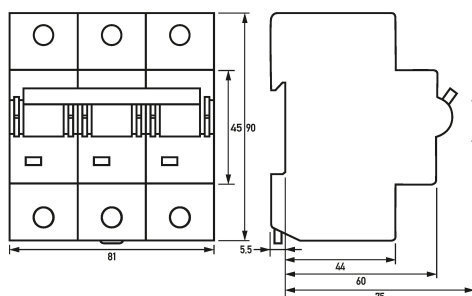
Dibujo acotado Interruptores magnetotérmicos DMCB 2 Co63-3
