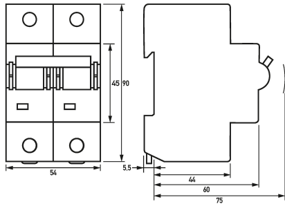
Dibujo acotado Interruptores magnetotérmicos DMCB 2 C100-2
