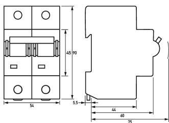
Maßzeichnung Gruppenansicht
