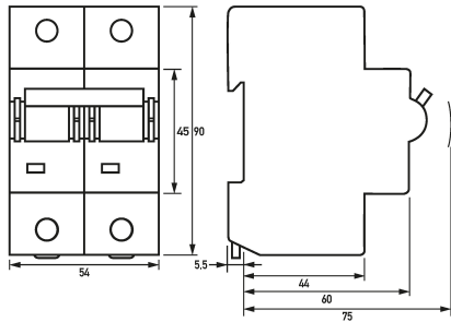
Dibujo acotado Interruptores magnetotérmicos DMCB 2 Co80-2
