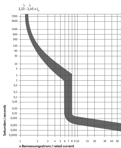
Diagramas Interruptores magnetotérmicos DMCB 2 C125-1
