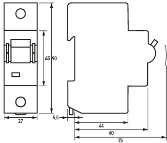
Dibujo acotado Interruptores magnetotérmicos DMCB 2 C100-1
