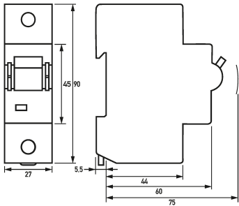
Dibujo acotado Interruptores magnetotérmicos DMCB 2 Co80-1
