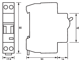
Maßzeichnung Leitungsschutzschalter ELS 3 C25/1+N
