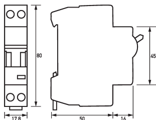
Maßzeichnung Leitungsschutzschalter ELS 3 Co6/1+N
