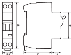
Dibujo acotado Vista de grupos
