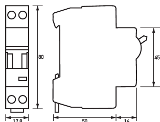
Dibujo acotado Interruptores magnetotérmicos ELS 3 B25/1+N
