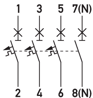
Esquema de conexiones DLS 6h, característica C, tres polos + N
