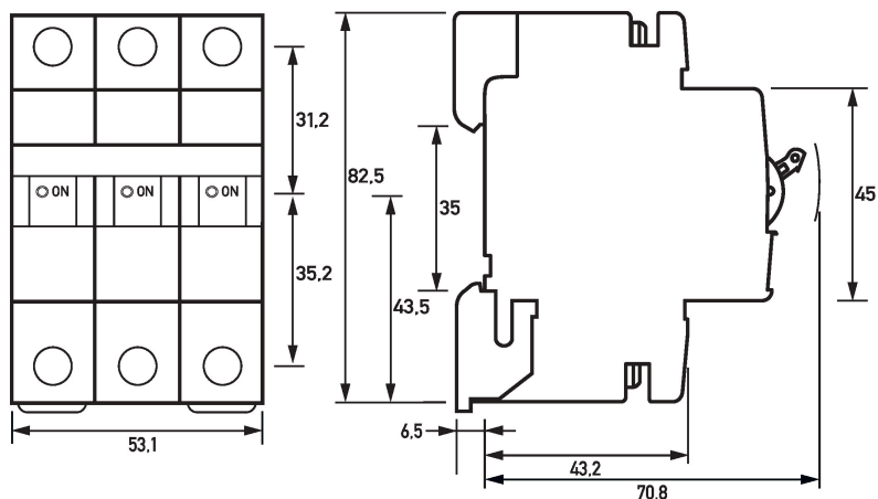
Dibujos acotados DLS 6h, característica C, tres polos (Vista de grupos)
