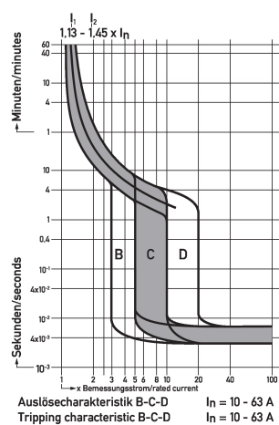
Curva característica Característica B, C, D
