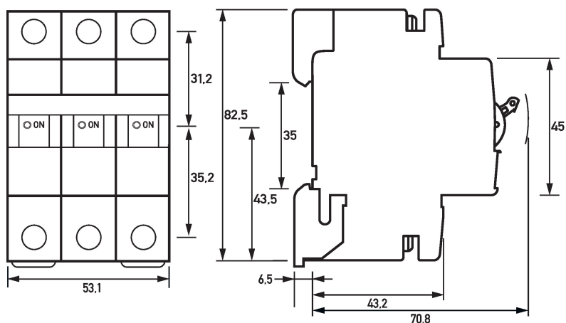
Dibujo acotado DLS 6h, característica C, tres polos (Vista de grupos)
