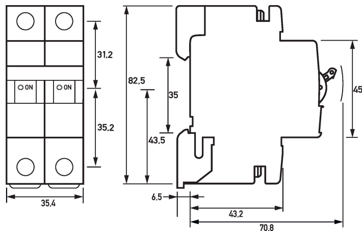
Dibujo acotado DLS 6h, característica C, dos polos (Vista de grupos)
