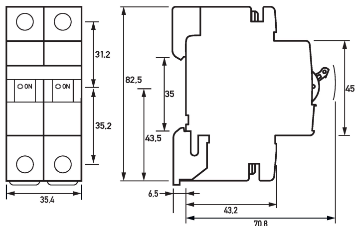
Dibujo acotado DLS 6h, característica C, un polo + N (Vista de grupos)
