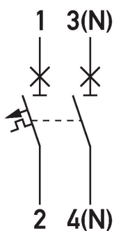
Anschlussschema DLS 6h, C-Charakteristik, einpolig+N
