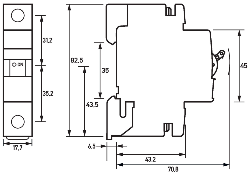
Dibujo acotado DLS 6h, característica C, un polo (Vista de grupos)
