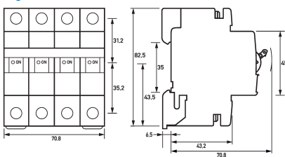
Maßzeichnung Gruppenansicht
