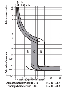
Curva característica Característica B, C, D
