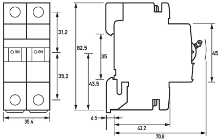
Dibujo acotado Interruptores magnetotérmicos DLS 6h B10-1+N
