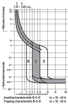
Diagramas Interruptores magnetotérmicos DLS 6h B10-1+N
