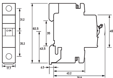
Dibujo acotado Interruptores magnetotérmicos DLS 6h, característica B
