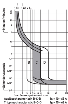
Diagramas Interruptores magnetotérmicos DLS 6h, característica B
