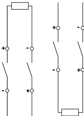
Ejemplo de cableado Interruptores magnetotérmicos DLS 6hdc B63-2
