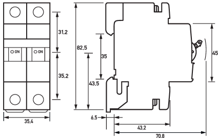
Dibujo acotado Interruptores magnetotérmicos DLS 6hdc B63-2
