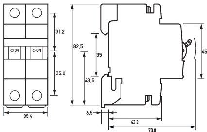
Dibujo acotado Interruptores magnetotérmicos DLS 6hdc B8-2
