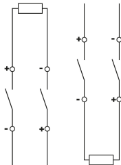
Ejemplo de cableado Interruptores magnetotérmicos DLS 6hdc B8-2
