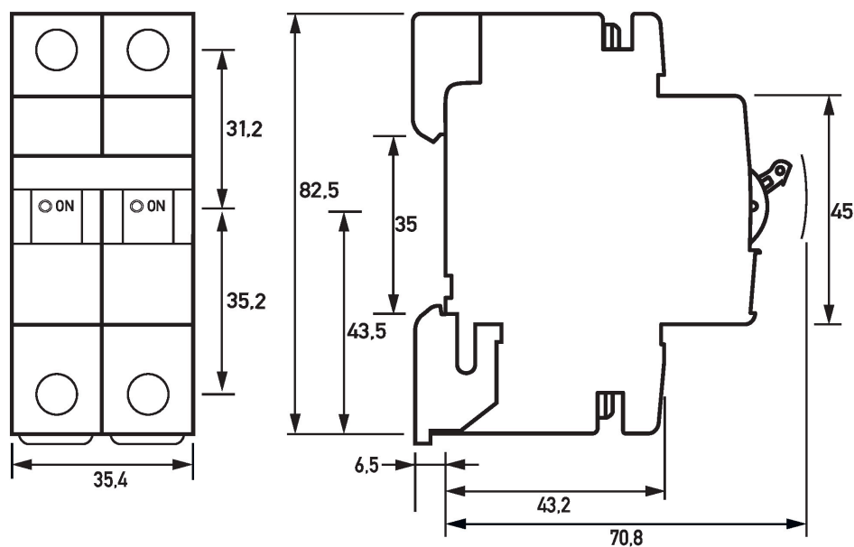
Dibujo acotado DLS 6hdc, característica B, dos polos (Vista de grupos)
