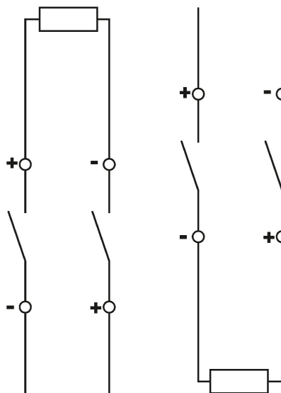
Esquema de conexiones DLS 6hdc, característica B, dos polos
