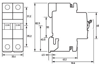
Maßzeichnung Gruppenansicht
