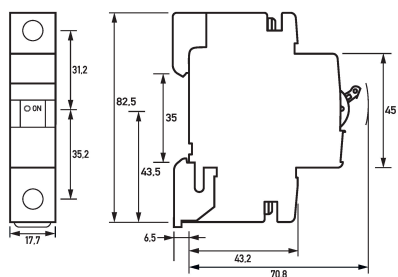
Maßzeichnung Leitungsschutzschalter DLS 6hdc B32-1
